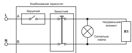
Рис. 6. Схема електрична
